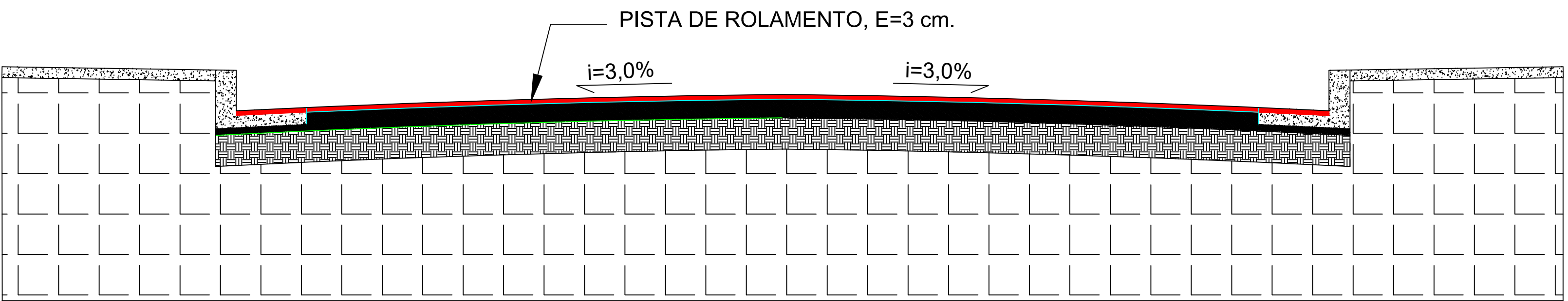
CORTE NA SEÇÃO TRANSVERSAL TRECHO DE 3 CM.
