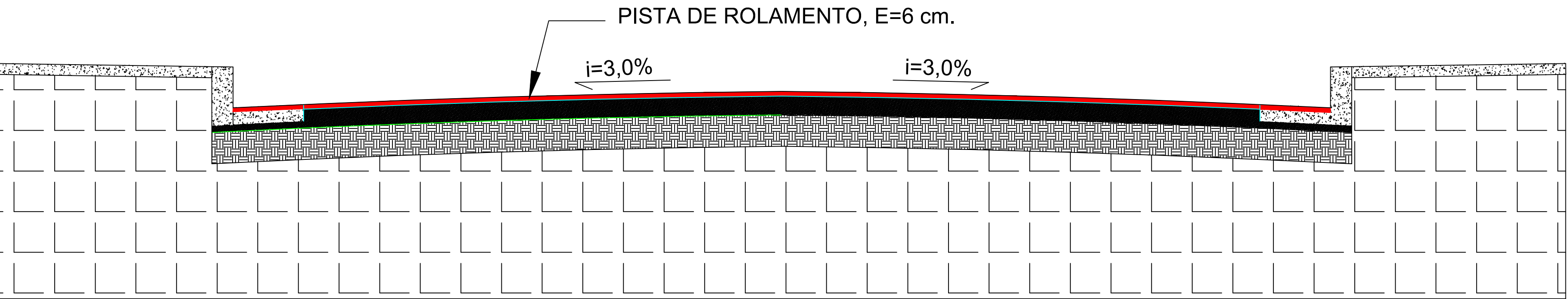
CORTE NA SEÇÃO TRANSVERSAL TRECHO DE 6 CM
